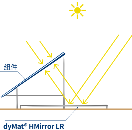
双面组件的改装
